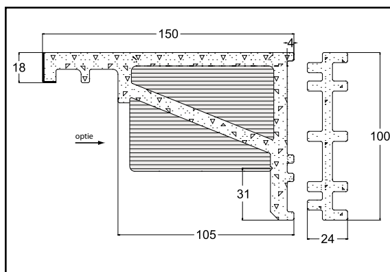
Beglaasde montage mogelijk met Recyclick montage systeem.
