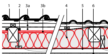
Naderhand aangebrachte isolatie tussen de dakspanten
