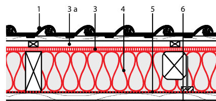
Isolatie tussen de dakspanten (nieuwbouw)
