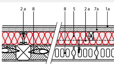
Buitenmuur massiefbouw
