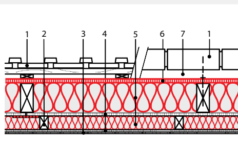
Buitenmuur lage energiewoning (houtspantenbouw)
